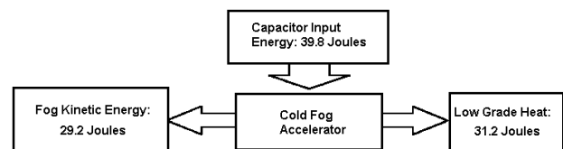
Fig. 1. Cold Fog Energy Flow
